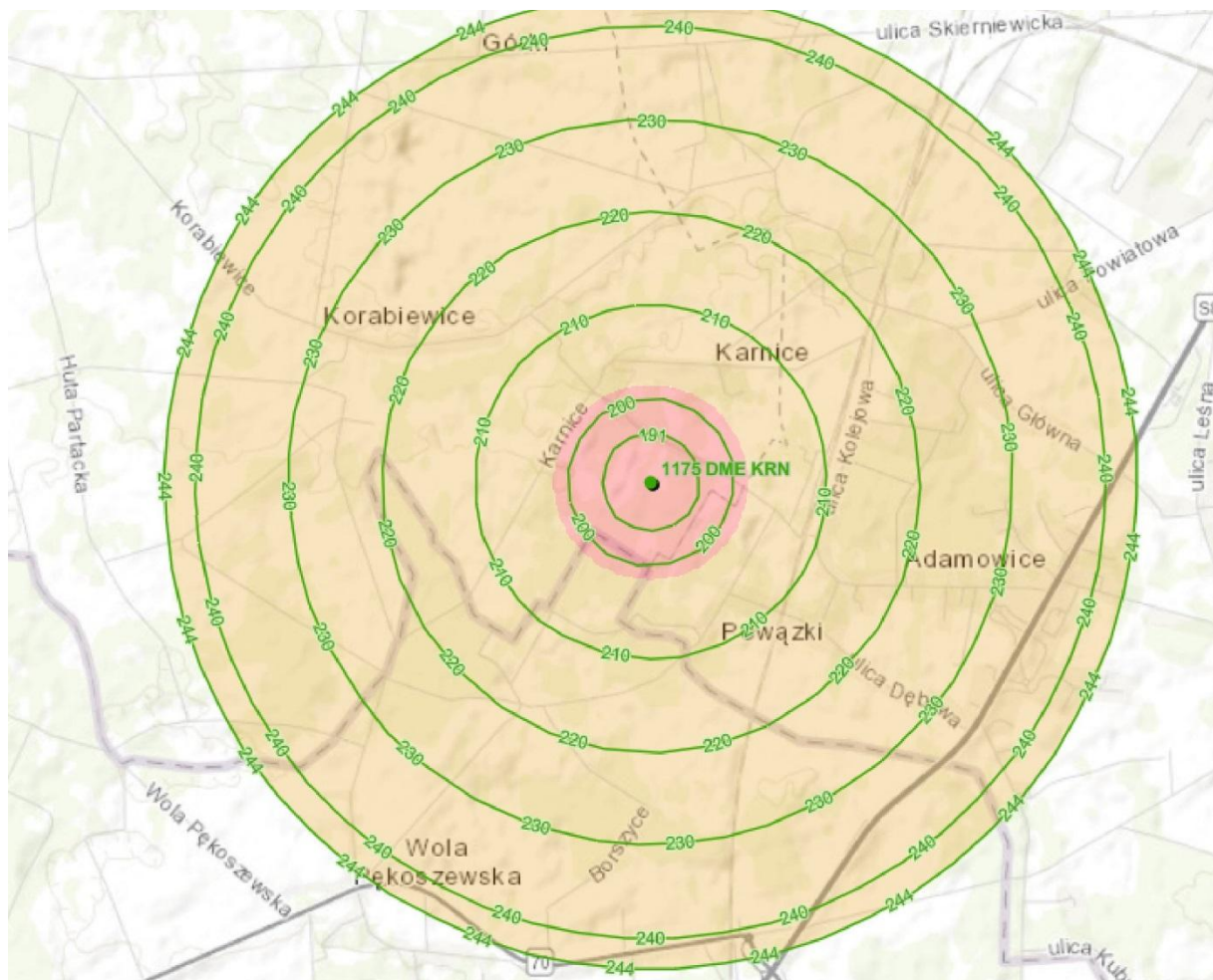
Mapa nr 5 Wizualizacja powierzchni ograniczających zabudowę (BRA) od punktu 1175 DME KRN w Karnicach Źródło: opracowanie własne na podstawie danych z Urzędu Lotnictwa Cywilnego ( www.ulc.gov.pl )
